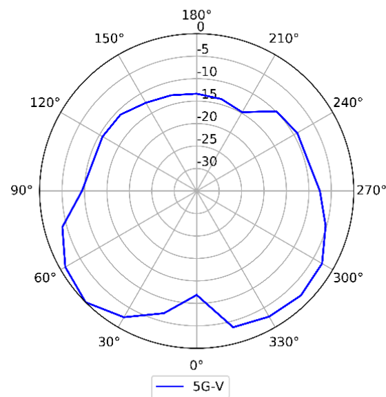
5GHz (Vertical)
