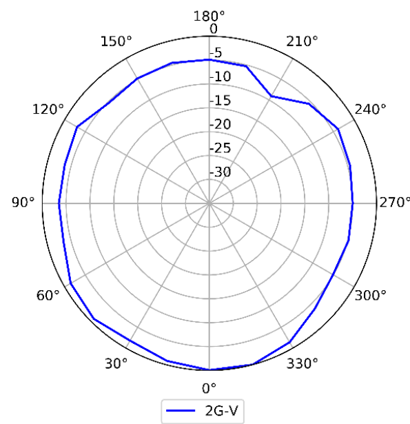
2.4GHz (Vertical)
