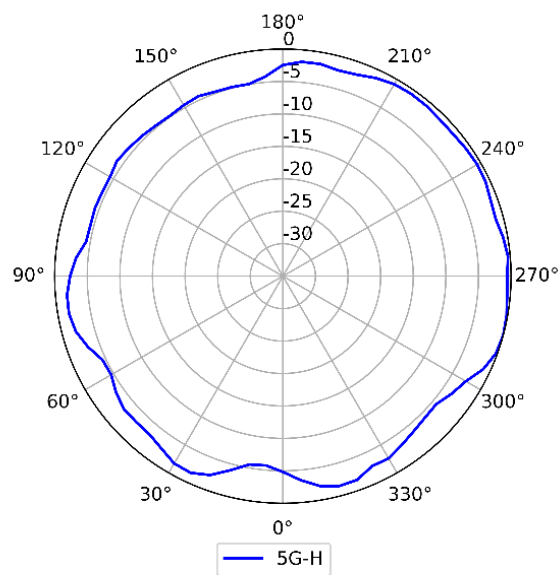
5GHz (Horizontal)
