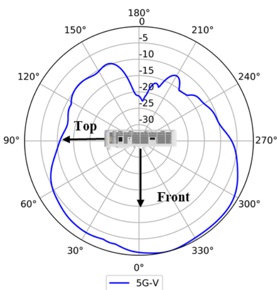
5GHz (Vertical)
