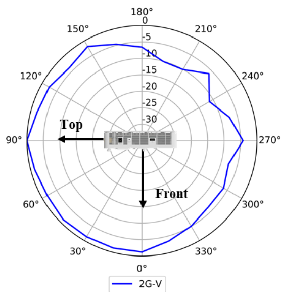
2.4GHz (Vertical)
