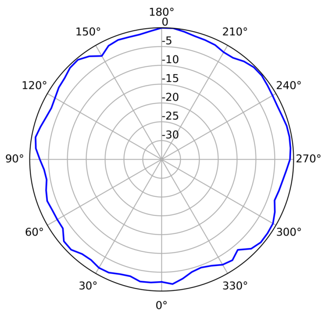
5GHz (Horizontal)
